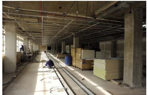
Colocación de bandejas de piso en el Edificio Rojo - Ministerio.
